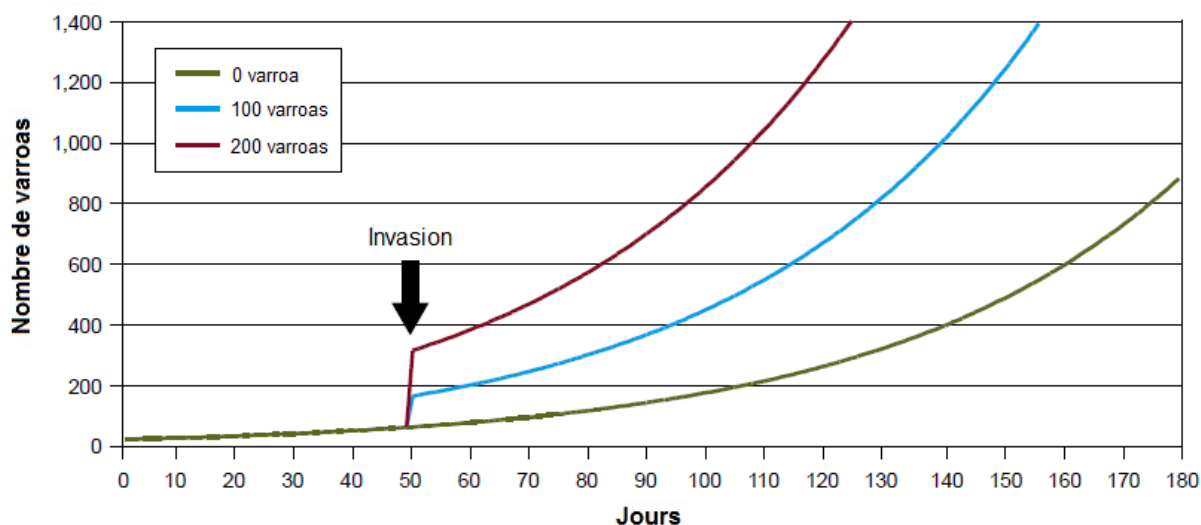
Figure 2. Modélisation de l'effet de l'apport de nouveaux varroas sur l'évolution du nombre de parasites au sein d'une colonie d'abeilles. Lorsqu'une colonie est initialement peu parasitée et en absence d'invasion par des varroas exogènes, la population de varroas sera maintenue sous le seuil critique d'infestation (1 000 à 3 000 varroas). Par contre, l'invasion d'une colonie par de nouveaux acariens peut conduire à des niveaux d'infestation suffisamment élevés pour menacer la survie de cette colonie (selon le nombre d'acariens exogènes introduits). Figure adaptée de The National Bee Unit (2017).
